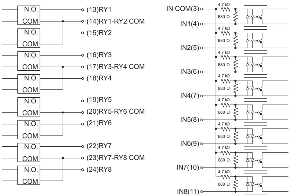
端子台连接图
