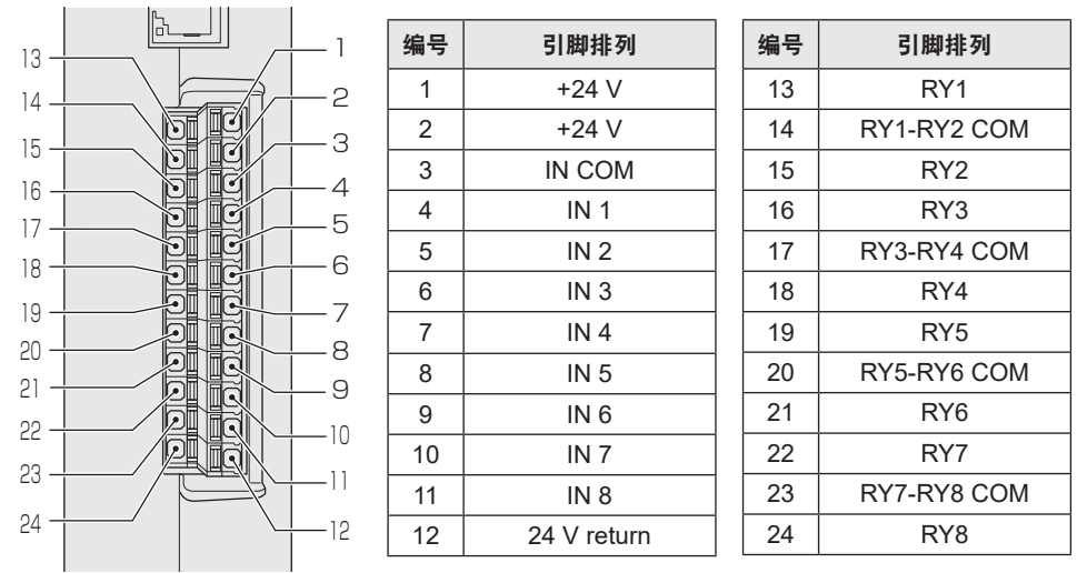
输出继电器和输入端子的分配
