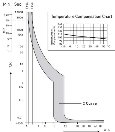
Karakteristik Kurva
